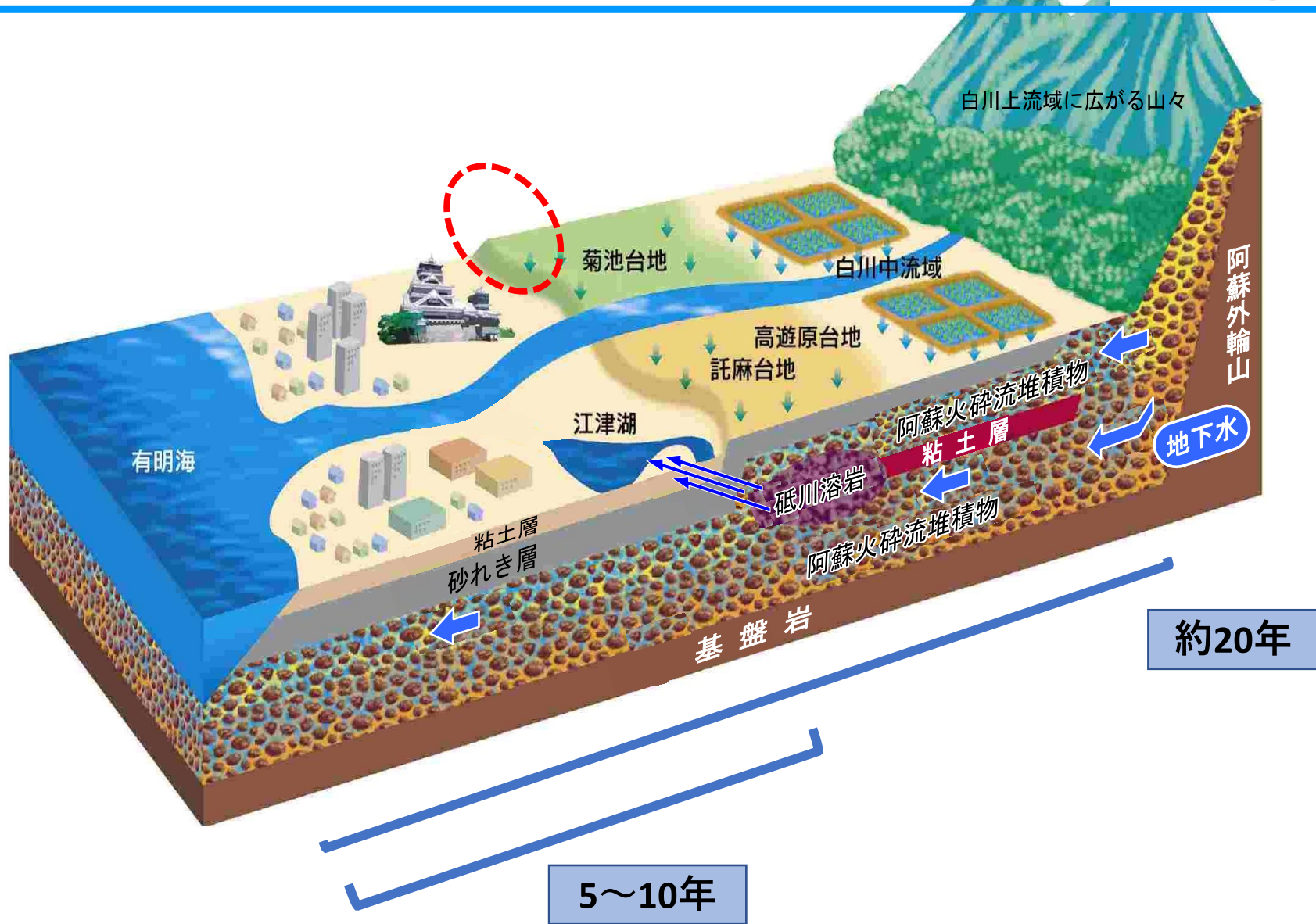
熊本地域の地下水の流れ
